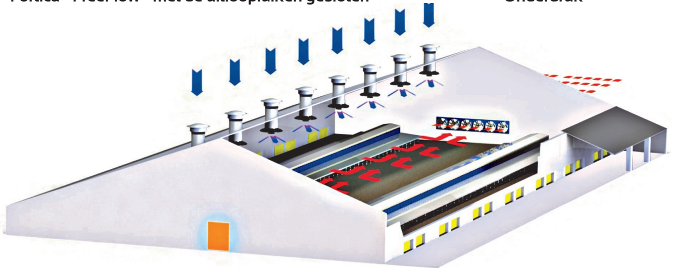
Fortica® FreeFlow® met de uitloopluiken gesloten
